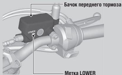
Передний тормоз
