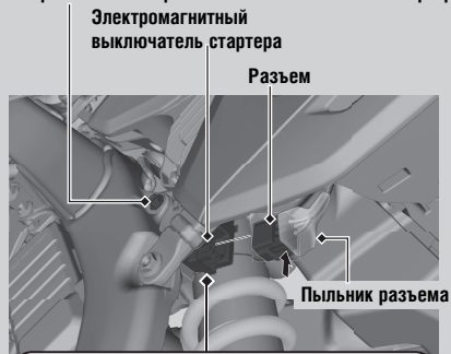
Запасной главный предохранитель (Spare main fuse) and Крышка электромагнитного выключателя стартера (Starter solenoid cover)
